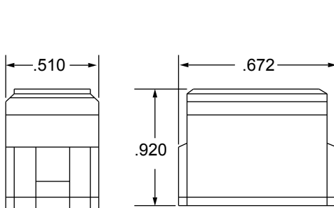
CTD16 Module
